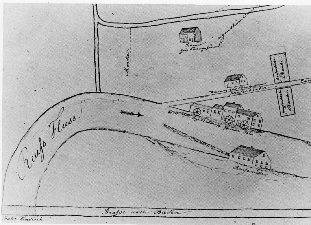
Planskizze, die dem Konzessionsgesuch von 1828 beigelegt wurde.
